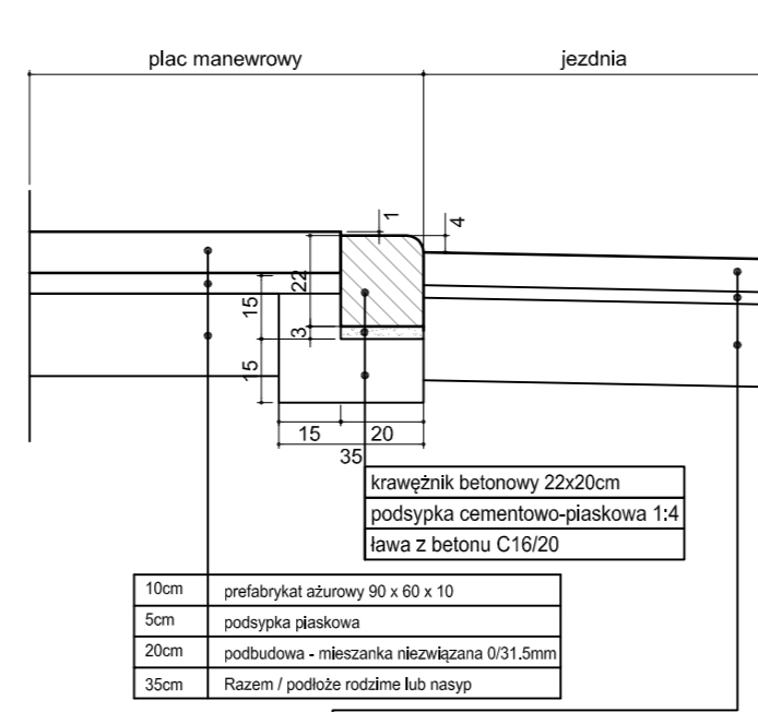
Szczegół "E" Krawężnik między jezdnią a placem manewrowym
