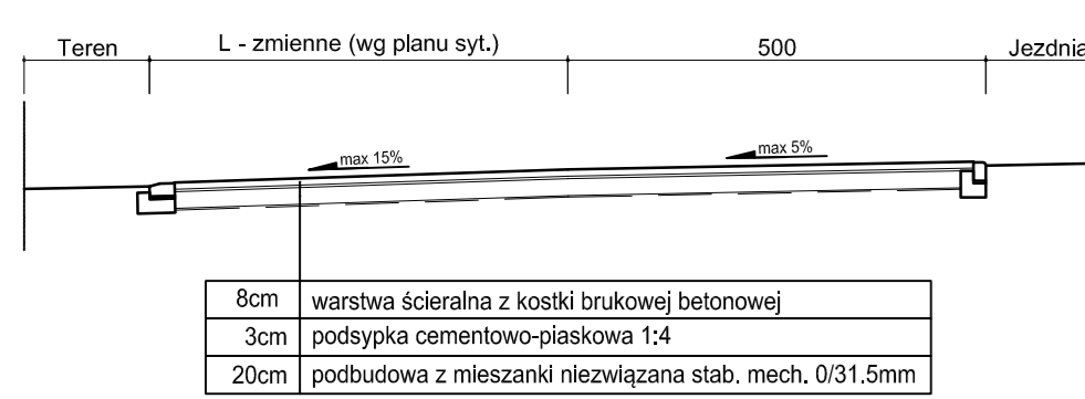
PRZEKRÓJ 1-1 SKALA 1:100
