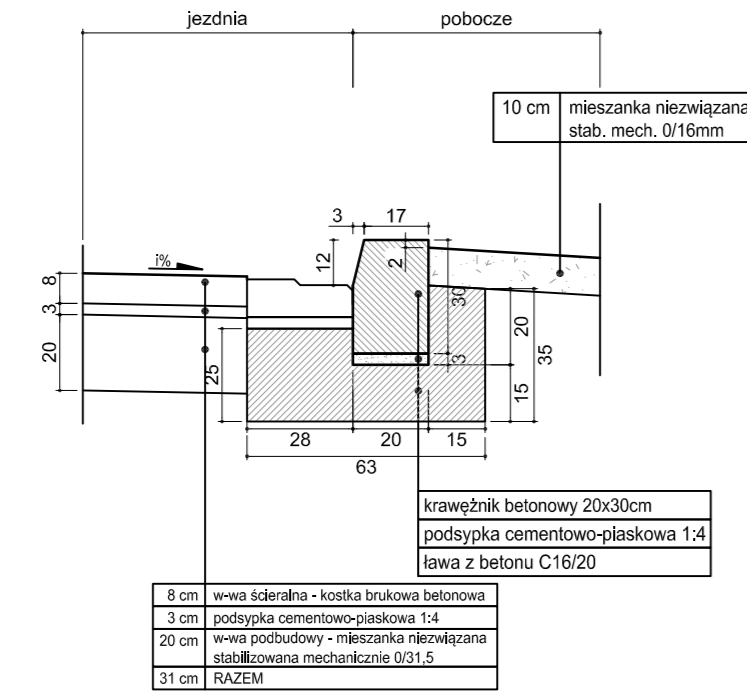
Szczegół "A" Krawężnik między jezdnią a poboczem ze ściekiem
