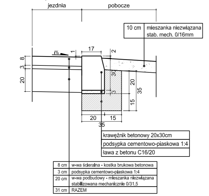
Szczegół "D" Krawężnik między jezdnią a poboczem bez ścieku
