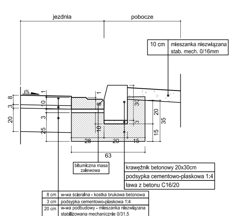
Szczegół "B" Ściek drogowy wibroprasowany
