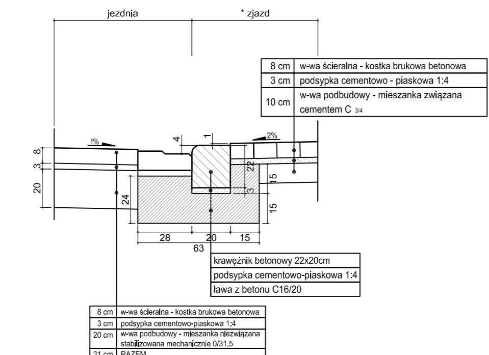
Szczegół "C" Krawężnik obniżony na zjazdach
